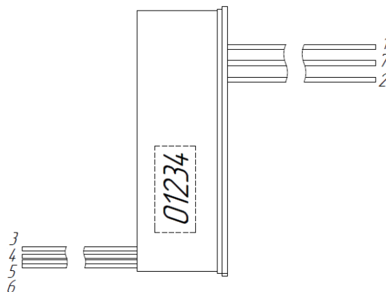
Рисунок 1. Расположение выводов
