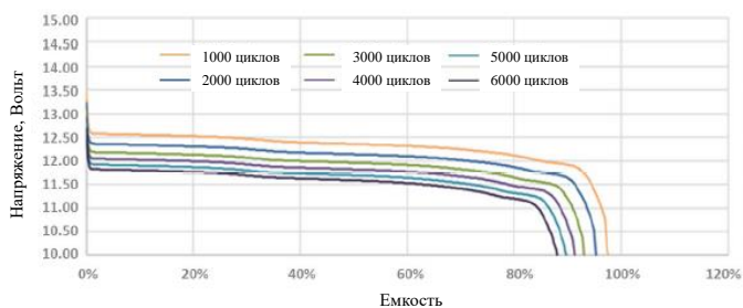
График разряда при глубине разряда 80% после различного числа рабочих циклов (стандартный заряд током 0,5С)
