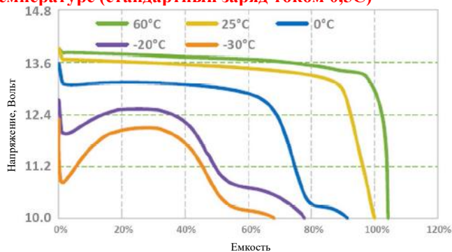
График разряда током 0,5С при различной температуре (стандартный заряд током 0,5С)
