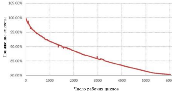
График степени заряда и разряда током 0,5С в зависимости от количества пережитых рабочих циклов
